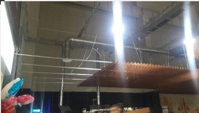
ТРЦ "Космополіт". Виготовлення та монтаж підвісної кубоподібної стелі загальною площею 320м 2 у приміщенні кафе та у тамбурах ТЦ «МегаМаркет»
